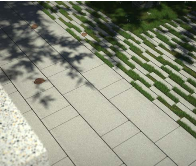
Strike 22x7,3 cm Classic Grijs in 'om en om verband' Flex Fusion Classic Grijs: 22x11 cm, 22x22 cm, 44x22 cm.
